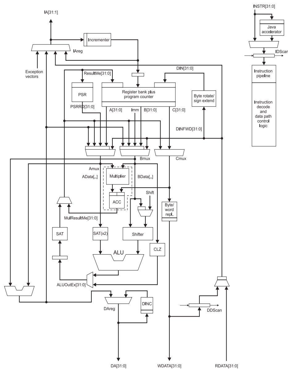
Σχήμα 2.1: Διάγραμμα Αρχιτεκτονικής
