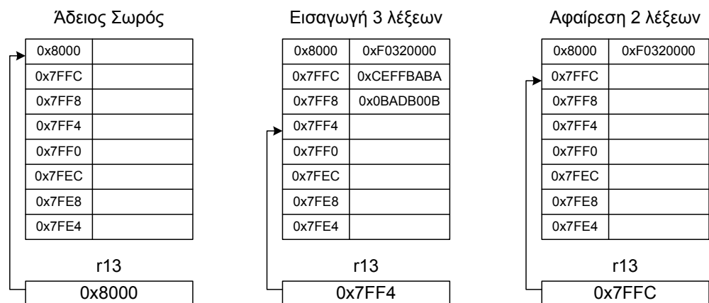
Σχήμα 2.4: Παράδειγμα σωρού.
