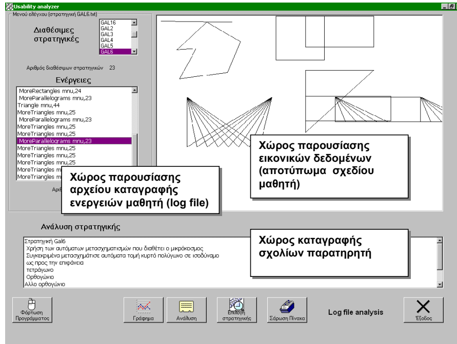
Εικόνα 4. Το περιβάλλον ανάλυσης δεδομένων πεδίου Usability Analyzer
